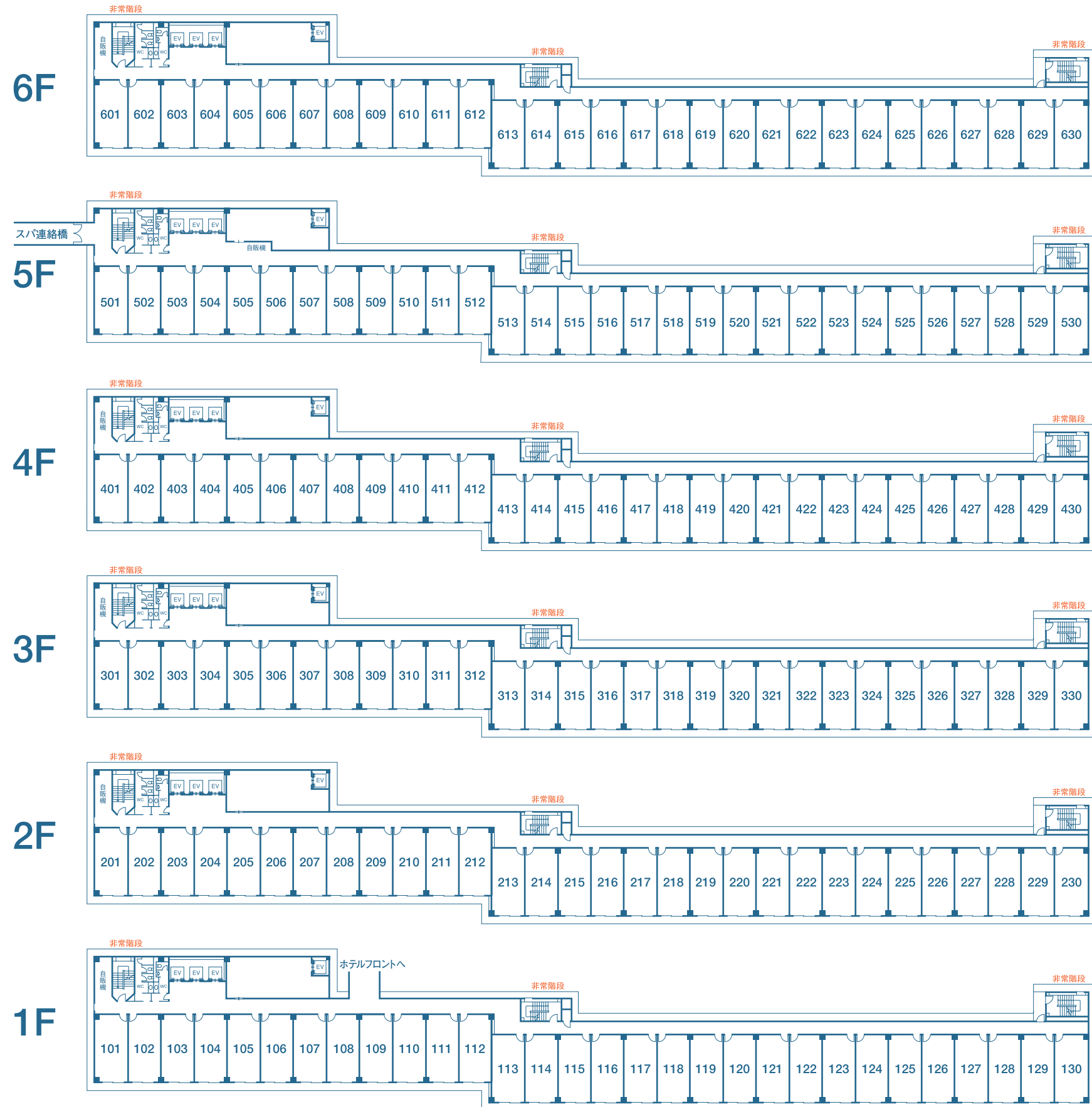
●基準室 1F~6F
